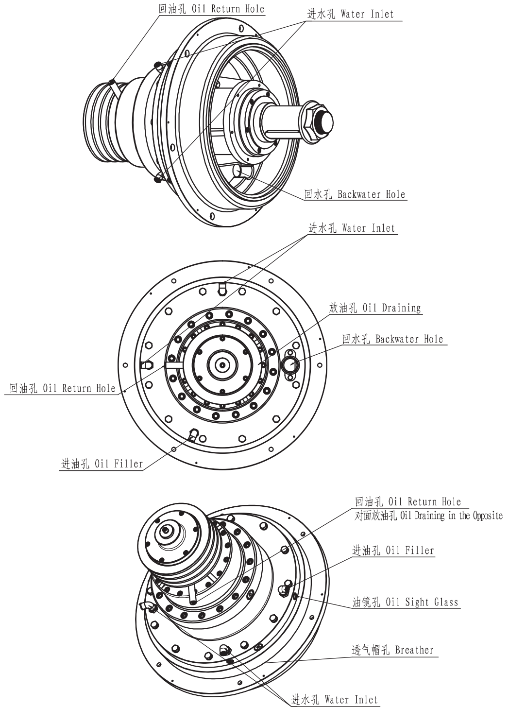
注油接水孔示意图 Oiling-Water Filler Sketch
